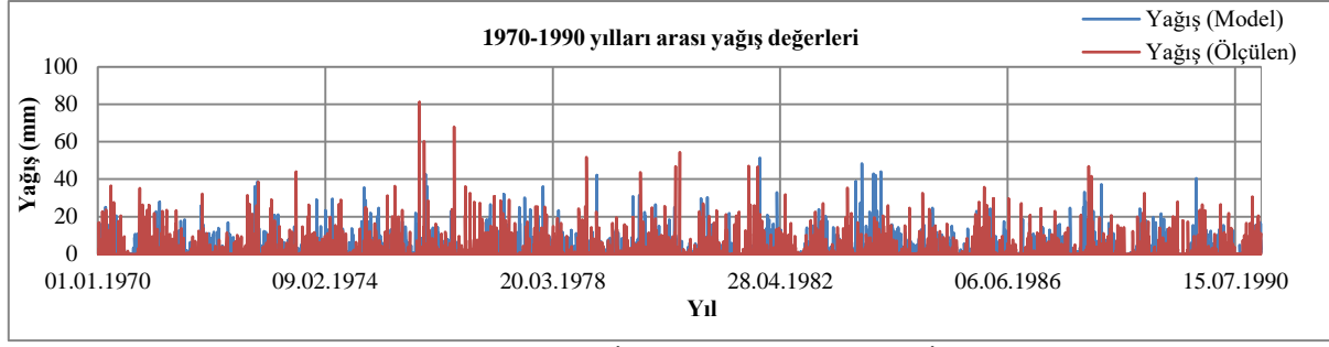
Şekil 5. 1970-1990 yılları arası Çorlu Meteoroloji İstasyonu ve RegCM3 Bölgesel İklim Modeli yağış (mm) değerleri Figure 5. Corlu Meteorology Station and RegCM3 Regional Climate Model precipitation (mm) values between 1970-1990
