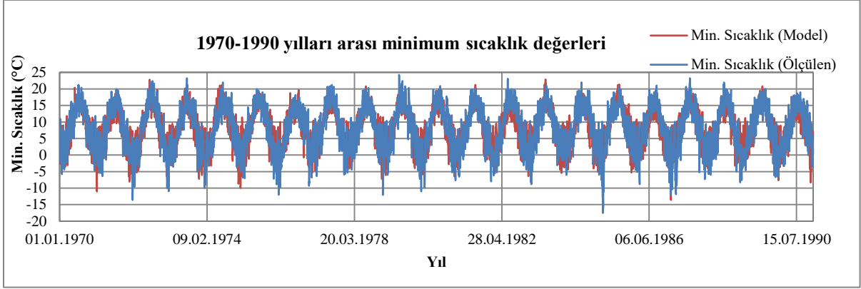
Şekil 2. 1970-1990 yılları arası Çorlu Meteoroloji İstasyonu ve RegCM3 Bölgesel İklim Modeli minimum sıcaklık (°C) değerleri Figure 2. Çorlu Meteorology Station and RegCM3 Regional Climate Model minimum temperature (°C) values
