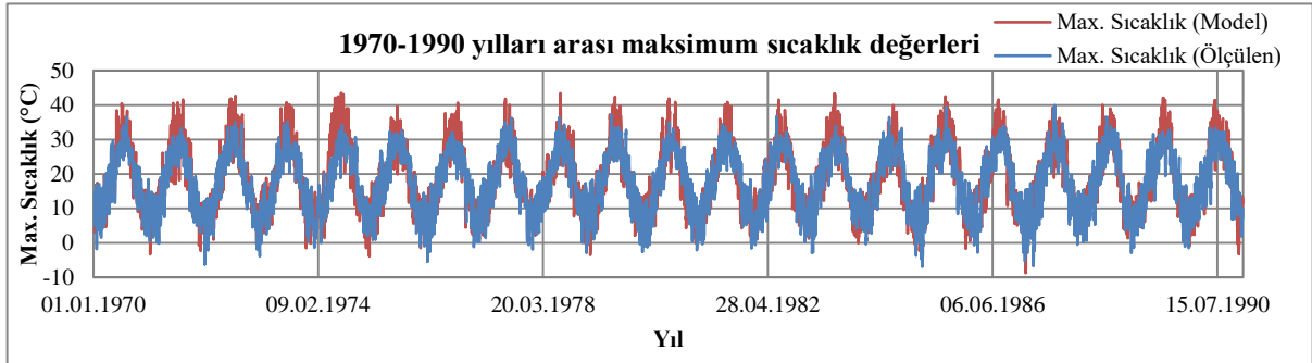
Şekil 3. 1970-1990 yılları arası Çorlu Meteoroloji İstasyonu ve RegCM3 Bölgesel İklim Modeli maksimum sıcaklık (°C) değerleri Figure 3. Çorlu Meteorology Station and RegCM3 Regional Climate Model maximum temperature (°C) values
